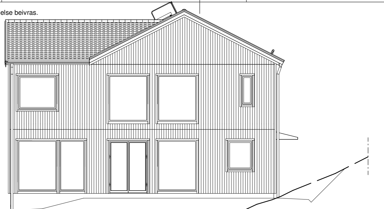
FASAD MOT SYDVÄST
